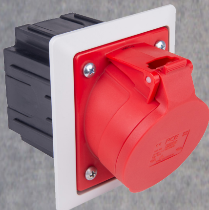
Gniazdo czerwone z puszką podtynkową i ramką 80 x 97mm, kołnierzyk jasnoszary, IP 44/54
